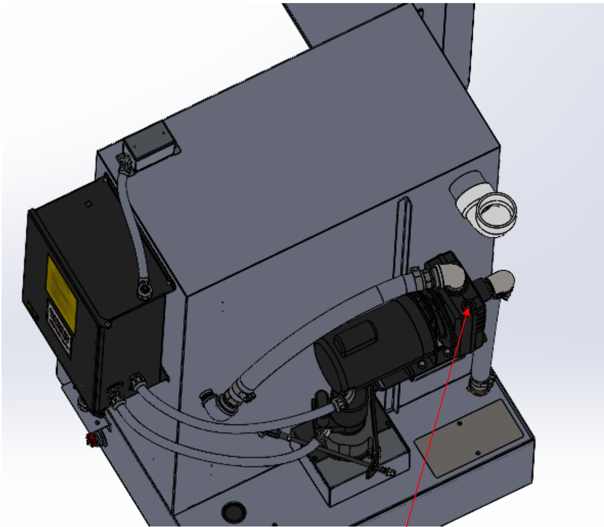
Pump Fill Port
